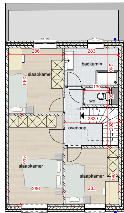
1e verdiep
