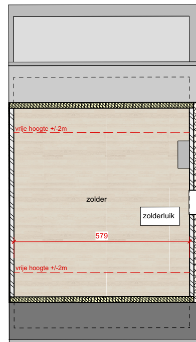
2e verdiep
